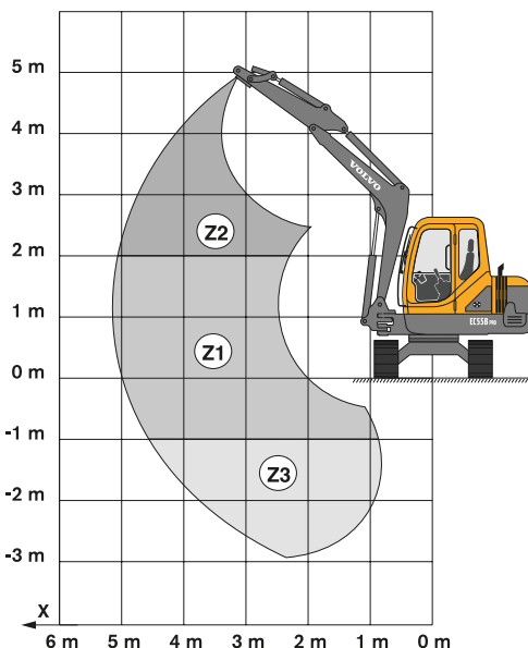
Løftkapacitet ved 360° drejning med bladet hævet.
